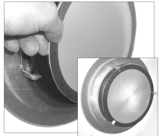
Einsetzen des Filtetägers: Zur Milderung des Hotspots Insert the filter holder: to alleviate the Hotspot
